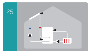
25 Солнечная установка с охлаждением 3 (охлаждение коллектора)
