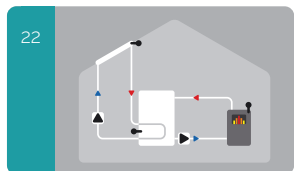
22 Солнечная установка с дровяным котлом
