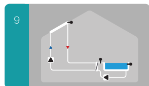
9 Солнечная установка с теплообменником (зонд на вторичном контуре) и бассейном
