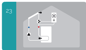
23 Солнечная установка с охлаждением 1 (охлаждение коллектора)
