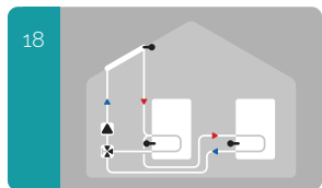
18 Солнечная установка с 2 накопителями и клапаном
