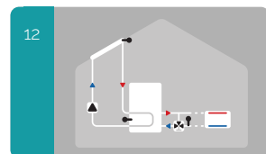
12 Солнечная установка с повышением температуры на обратной линии контура отопления
