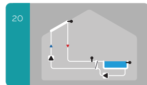
20 Солнечная установка с бассейном и теплообменником
