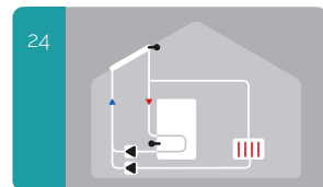
24 Солнечная установка с охлаждением 2 (охлаждение коллектора)
