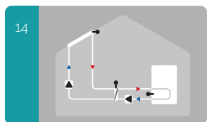
14 Солнечная установка с теплообменником
