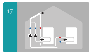
17 Солнечная установка с 2 накопителями и 2 насосами
