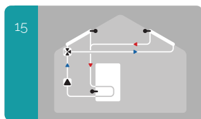
15 Солнечная установка с 2 коллекторами
