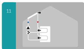
11 Солнечная установка с накопителем 2 зоны
