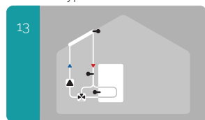
13 Солнечная установка с обходом
