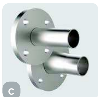
Trasformazione da attacco filettato in attacco flangiato
